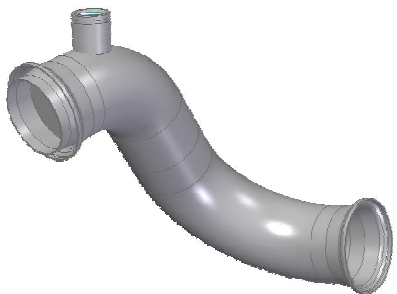
Tubo no kat - No kat pipe KT.020.C1
